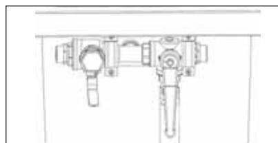
Påfyllnadspump i blandningssläge
